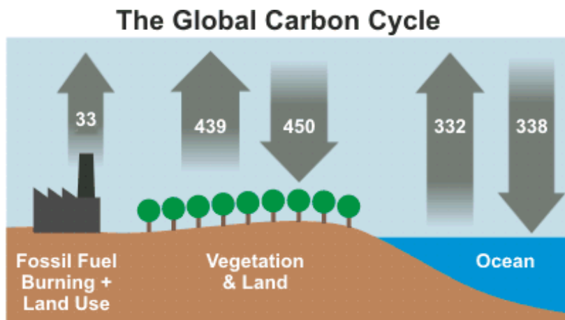
FIGUUR G WERELDWIJDE CO 2 BALANS IN GIGATON. BRON IPCC AR4. OPNAME EN UITSTOOT RESPECTIEVELIJK 788 EN 804 GIGATON.
