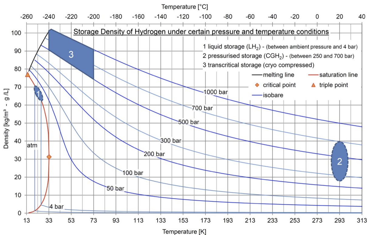
FIGUUR K RELATIE OPSLAGCAPACITEIT ALS FUNCTIE VAN TEMPERATUUR EN DRUK
