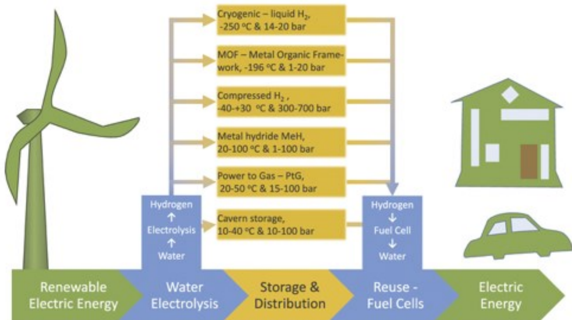
FIGUUR 0 DIVERSE MANIEREN OM WATERSTOF OP TE SLAAN BRON: ENGINEERING ENERGY STORAGE ODNE BURHEIM ISBN: 978-0-12-814100-7
