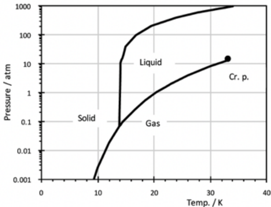
FIGUUR J FASE DIAGRAM WATERSTOF ALS FUNCTIE VAN DRUK EN TEMPERATUUR.
