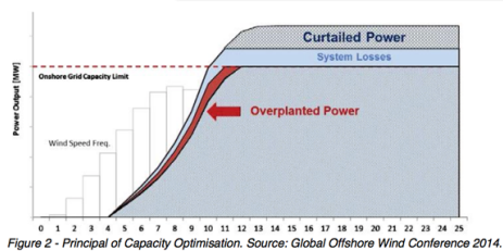
Figuur 2.5 Systemeverliezen, overplanting en curtailed power bij offshore park ontwerp
