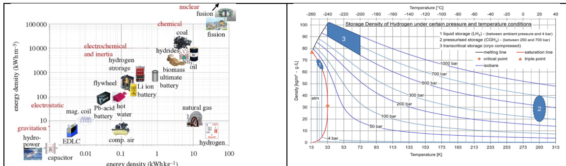
Figuur 2.1 energiedichtheid verschillende opslagsystemen en energiedichtheid waterstof bij verschillende druk en temperatuur
