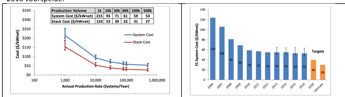
Figuur 2.11 Kostprijsontwikkeling brandstofcellen
