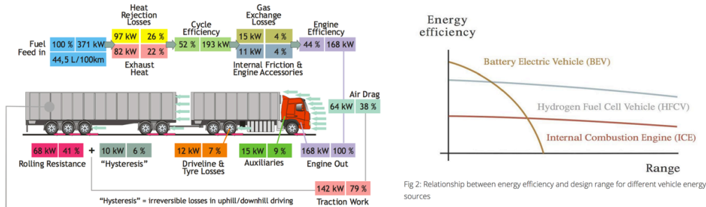
Figuur 2.13 energieverbruik vrachtwagen en voertuig efficiency
