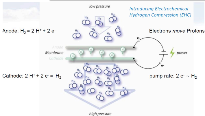
Figuur 2.4 Werkingsprincipe van Electro Chemische Compressie (CCC)
