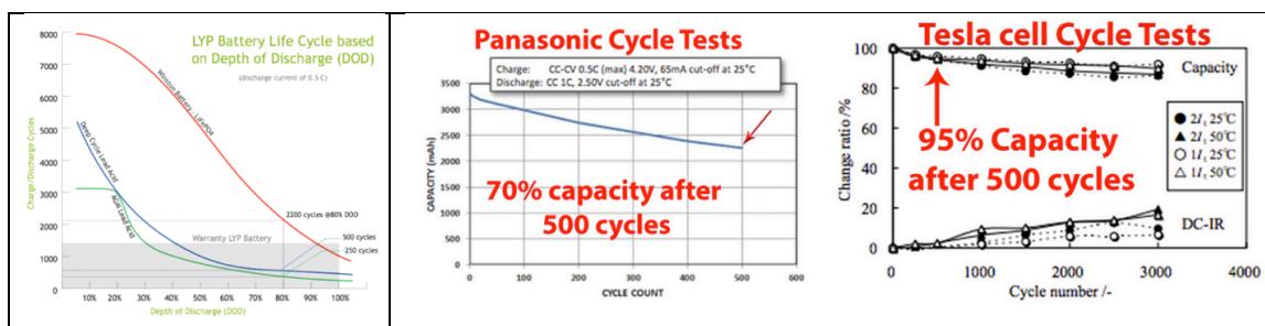
Figuur 2.14 levensduur en laadcycli batterijen
