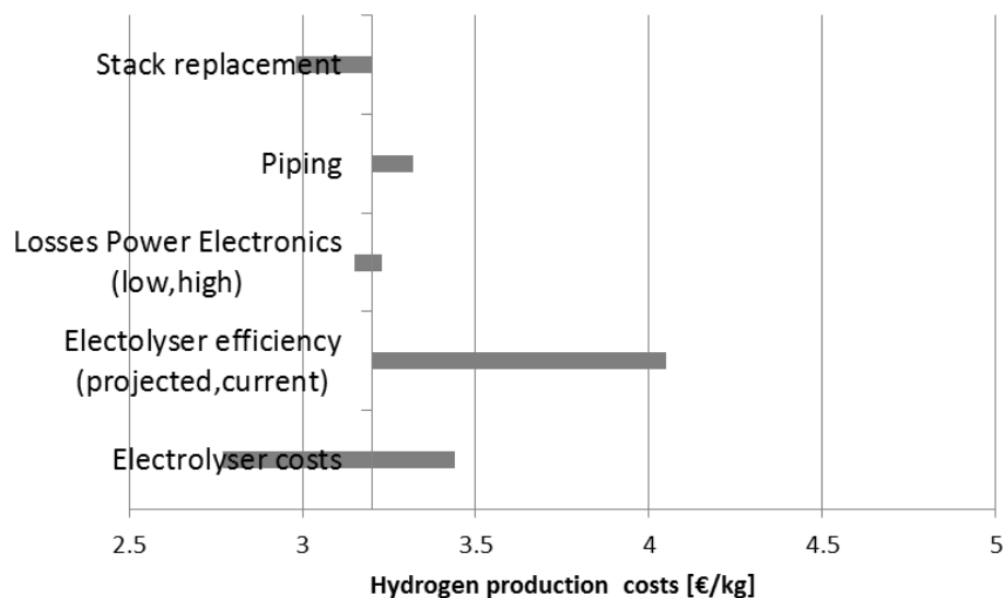
Figuur 2.7 Gevoeligheidsanalyse kostprijs waterstof uit offshore wind
